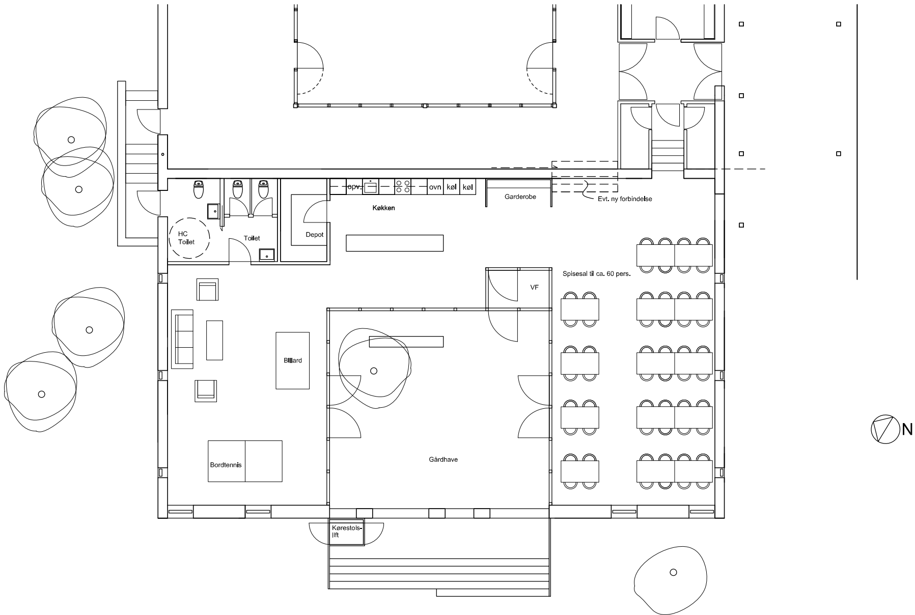
Plan fællesområde 1:100
